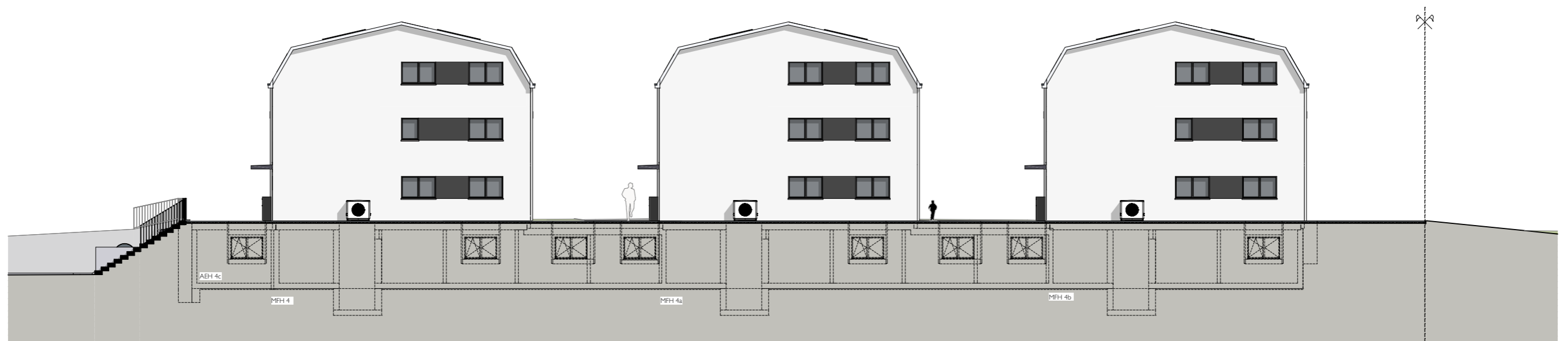
NORDFASSADE
