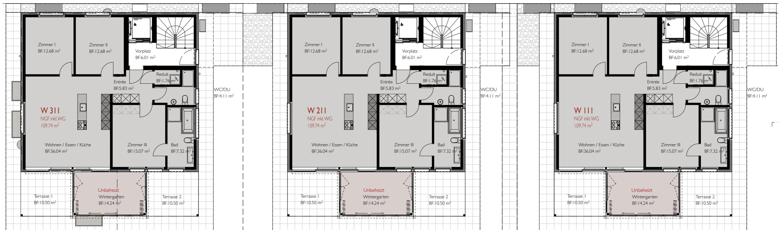
ERDGESCHOSS
