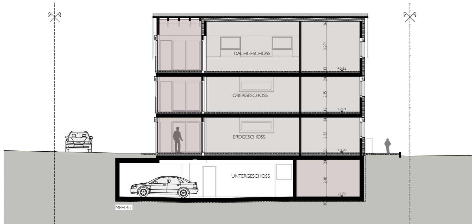
SCHNITT B-B
