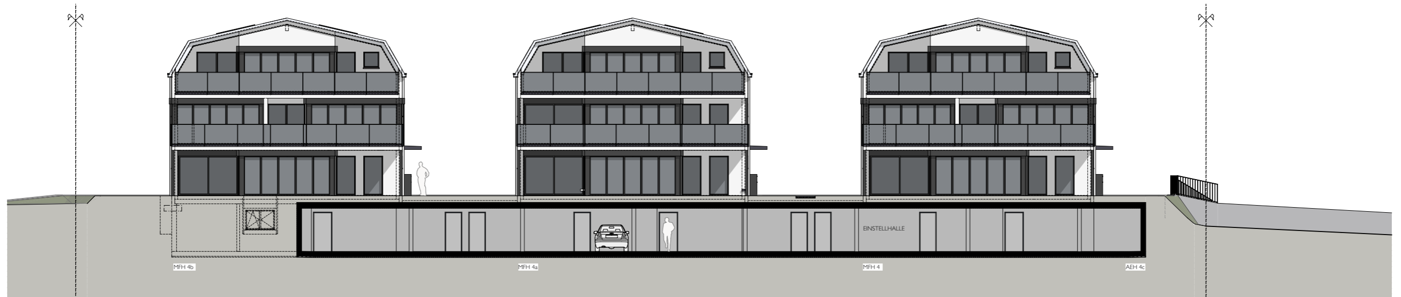
SÜDFASSADE
